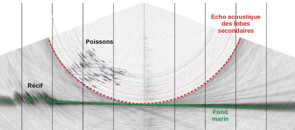
Figure 5. Exemple d'image de la colonne d'eau obtenue avec un sondeur multifaisceaux R2SONIC 2022.
