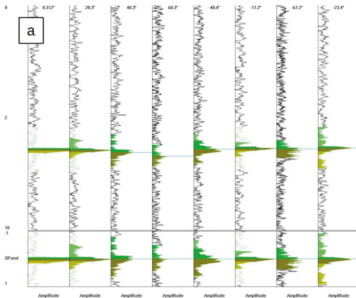
Figure 8. L'écho-intégration au sondeur multifaisceaux : a) analyse automatique du signal sur plusieurs faisceaux ; b) carte de l'écho-intégration d'un herbier sous-marin sur la partie ouest du Tombolo de Giens.
